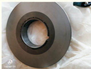
推力盘磨损图片
